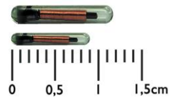
Puce électronique
